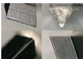
SIR0007K08CB (内部給油) 30 個加工後
